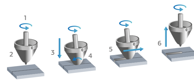
Der DynaSTIR Rührreibschweiß-Prozess
