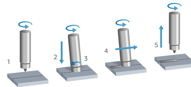
Der MonoSTIR Rührreibschweiß-Prozess
